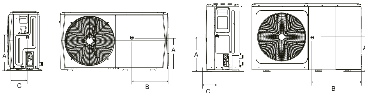
4/6 kW (unité : mm)
