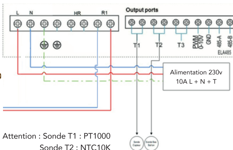
Câblage Régulation Solaire
